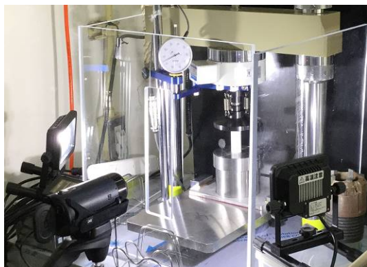
一軸圧縮強度測定
